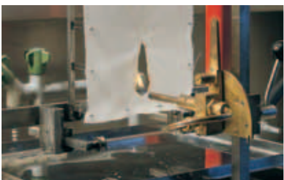
Für Brandversuche mit Dekostoffen wird dieser Kleinbrennertest nach der British-Standard-Norm BS 5438 eingesetzt.
